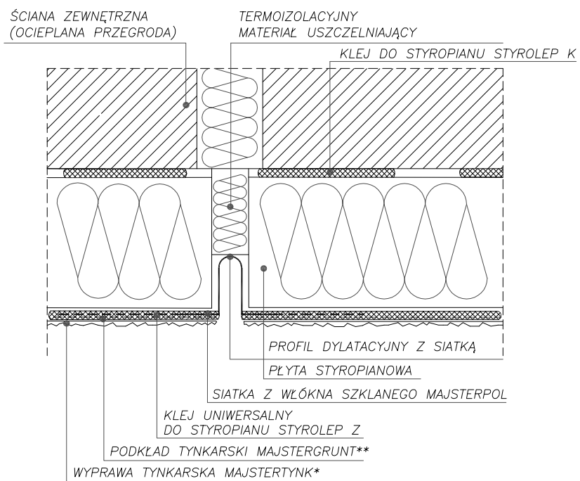
DETAL PRZERWY DYLATACYJNEJ PRZEKRÓJ POZIOMY
