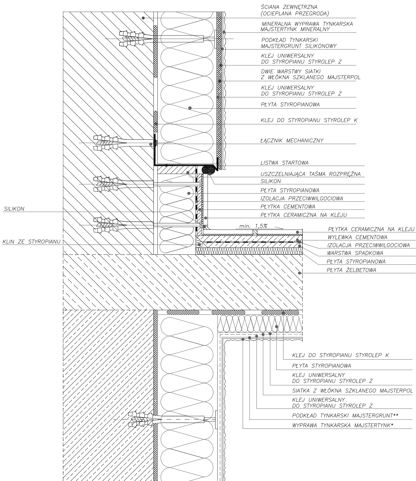
DETAL OCIEPLENIA ŚCIANY PRZY POŁĄCZENIU Z BALKONEM LUB LOGGIĄ PRZEKRÓJ POZIOMY
