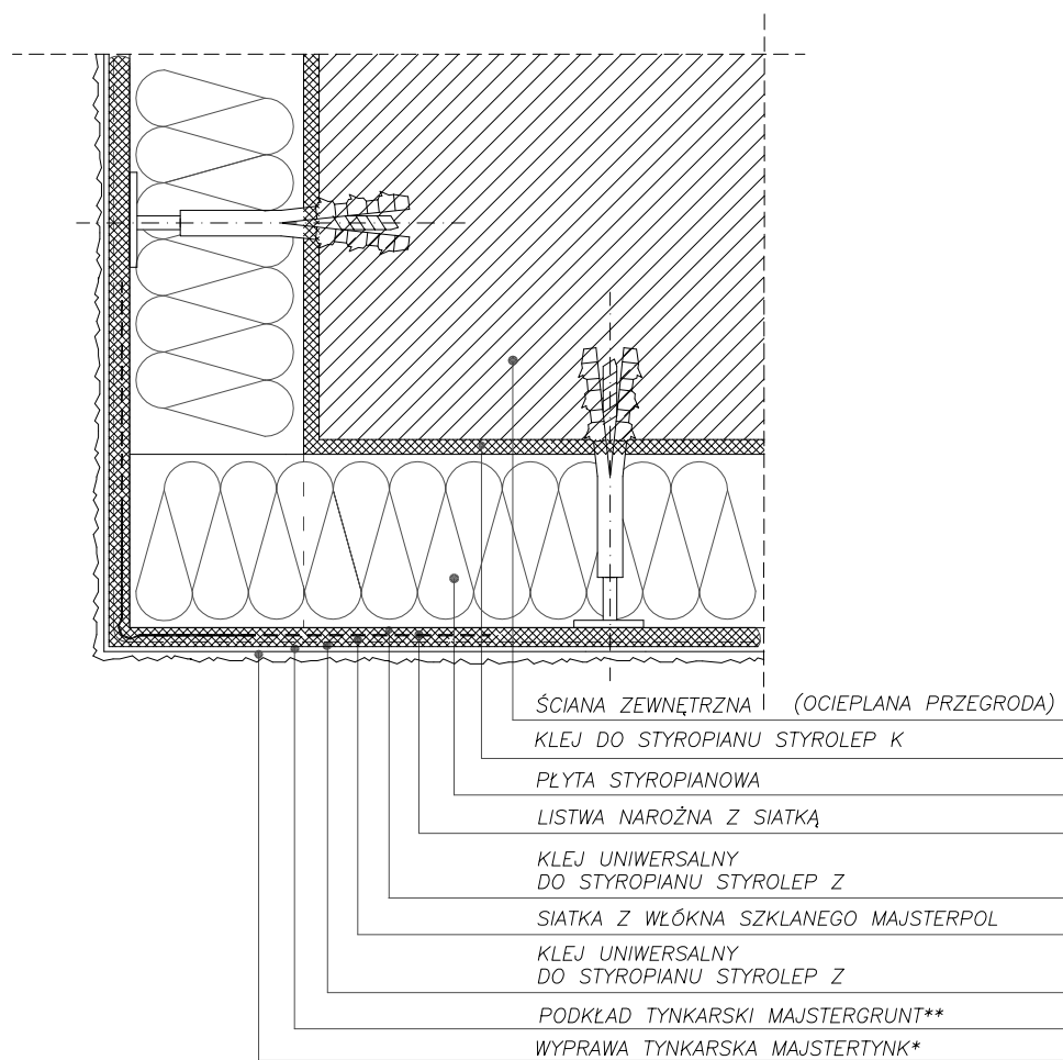
DETAL OCIEPLENIA NAROŻA WYPUKŁEGO PRZEKRÓJ POZIOMY
